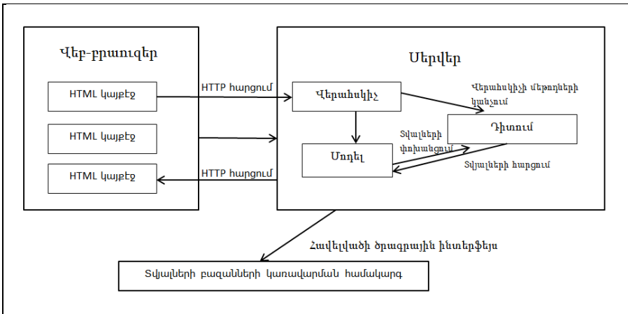
Նկար 1 . Դեղատնային ցանցում դեղերի որոնման տեղեկատվական համակարգի կառուցվածքը
