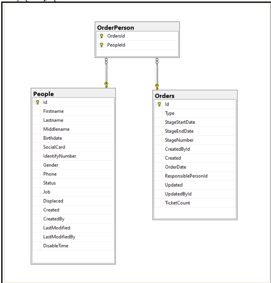
Նկար 1. Անձինք և Ստացականներ աղյուսակների միջև կապը
