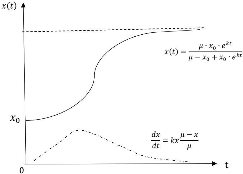
Նկար 1. Իրական պայմաններում պոպուլացիայի անդամների թվի (Լոգիստական կոր) և նրա փոփոխման արագության կախվածությունները ժամանակից
